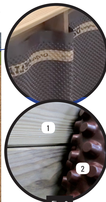
Fig. 6 1- Armação de madeira 2- Rolo de proteção e de drenagem alveolar de PEHD
