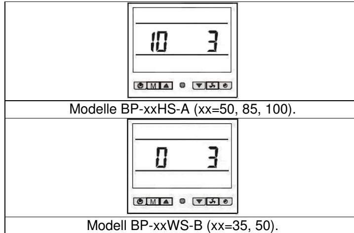
Abbildung 35: Programmierung des Parameters 10 (Parameter 0 beim Modell BP-xxWS-B (xx=35, 50)), Standardeinstellung.
