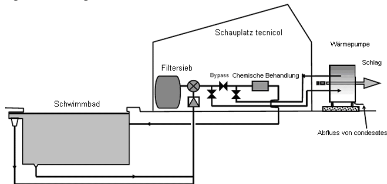
Abbildung 6: Typische Anordnung der Komponenten des Wasserkreislaufs.
