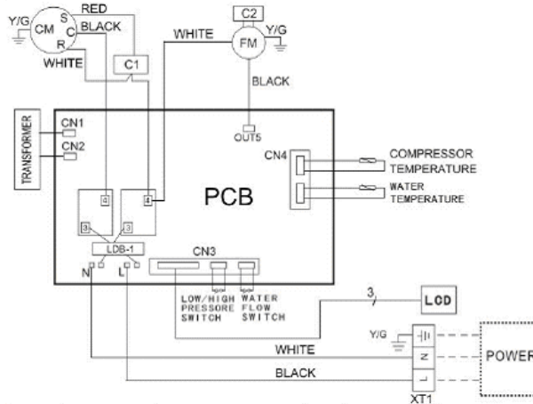
Abbildung 10: Schaltplan.
