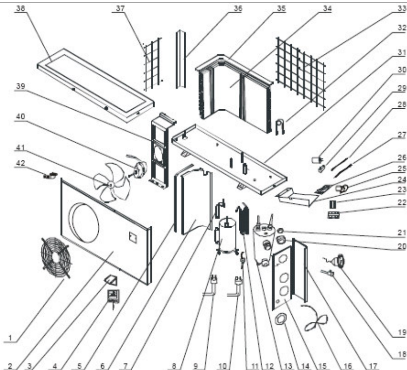
Abbildung 44: Explosionszeichnung der Ersatzteile.
