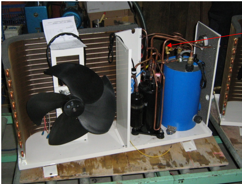
Abbildung 45: Ersetzung des Manometers.
