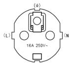
Abbildung 8: Illustration der am Stecker auszuführenden Anschlüsse.
